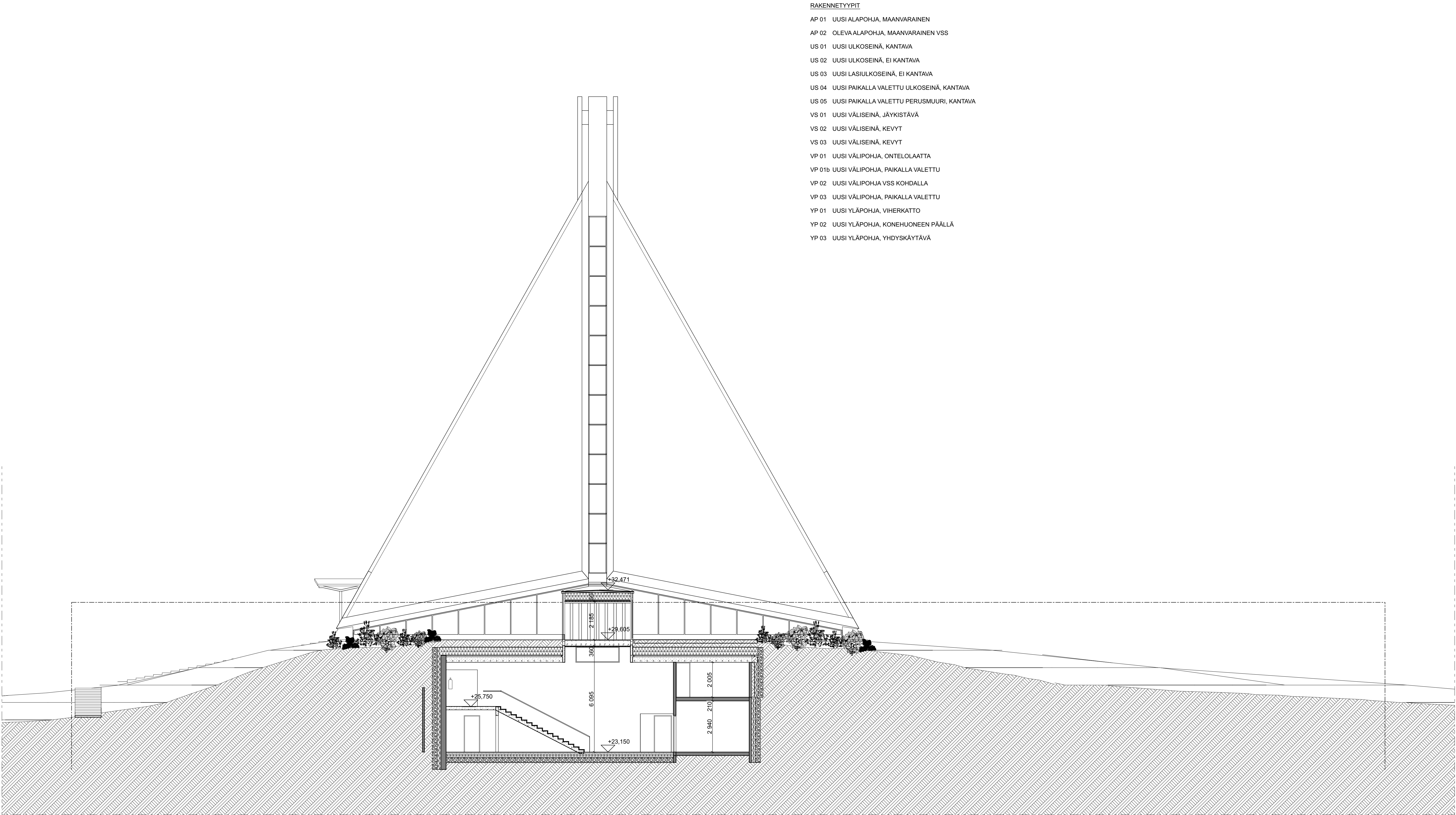
LEIKKAUS A-A
