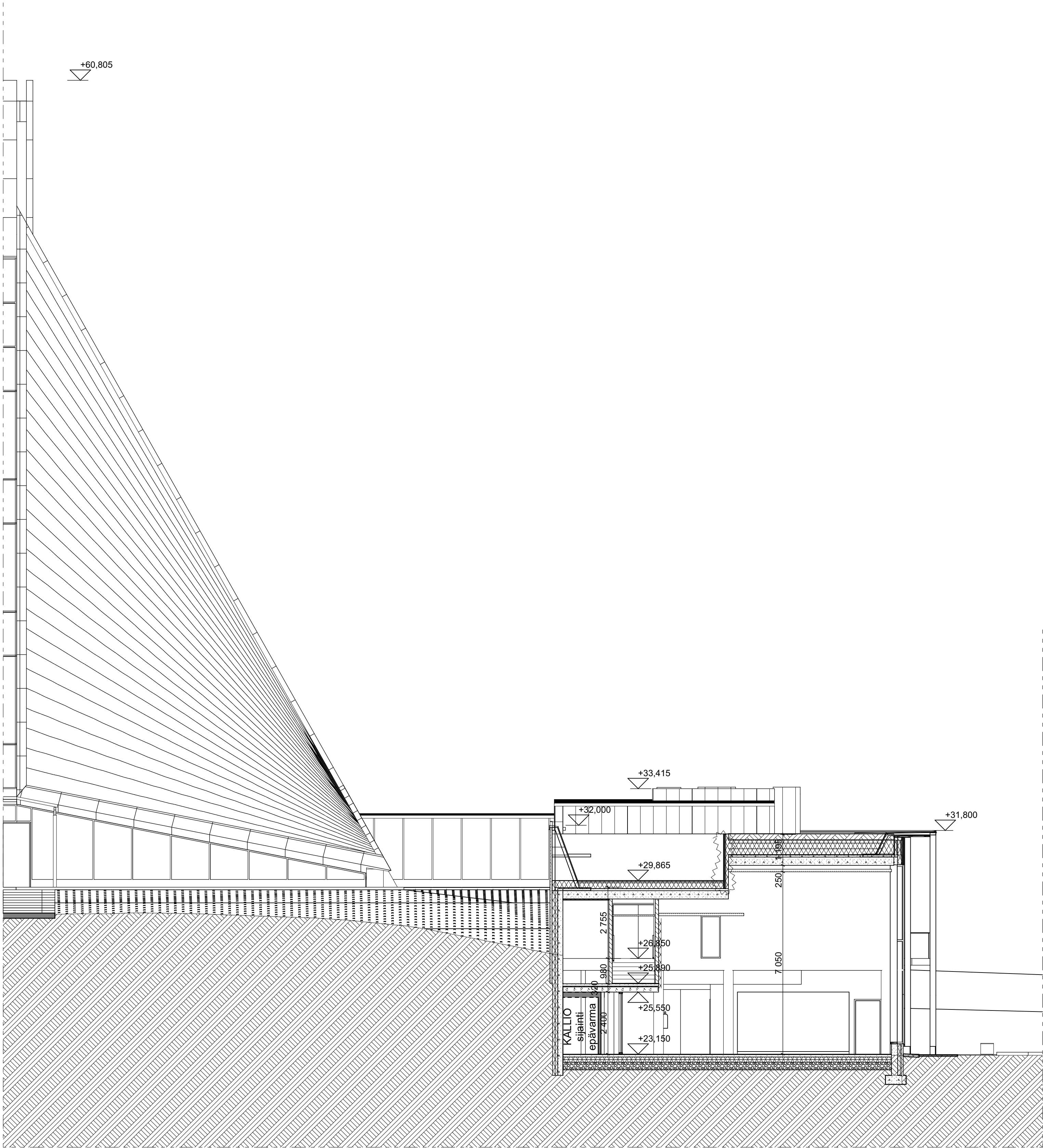
LEIKKAUS D-D
