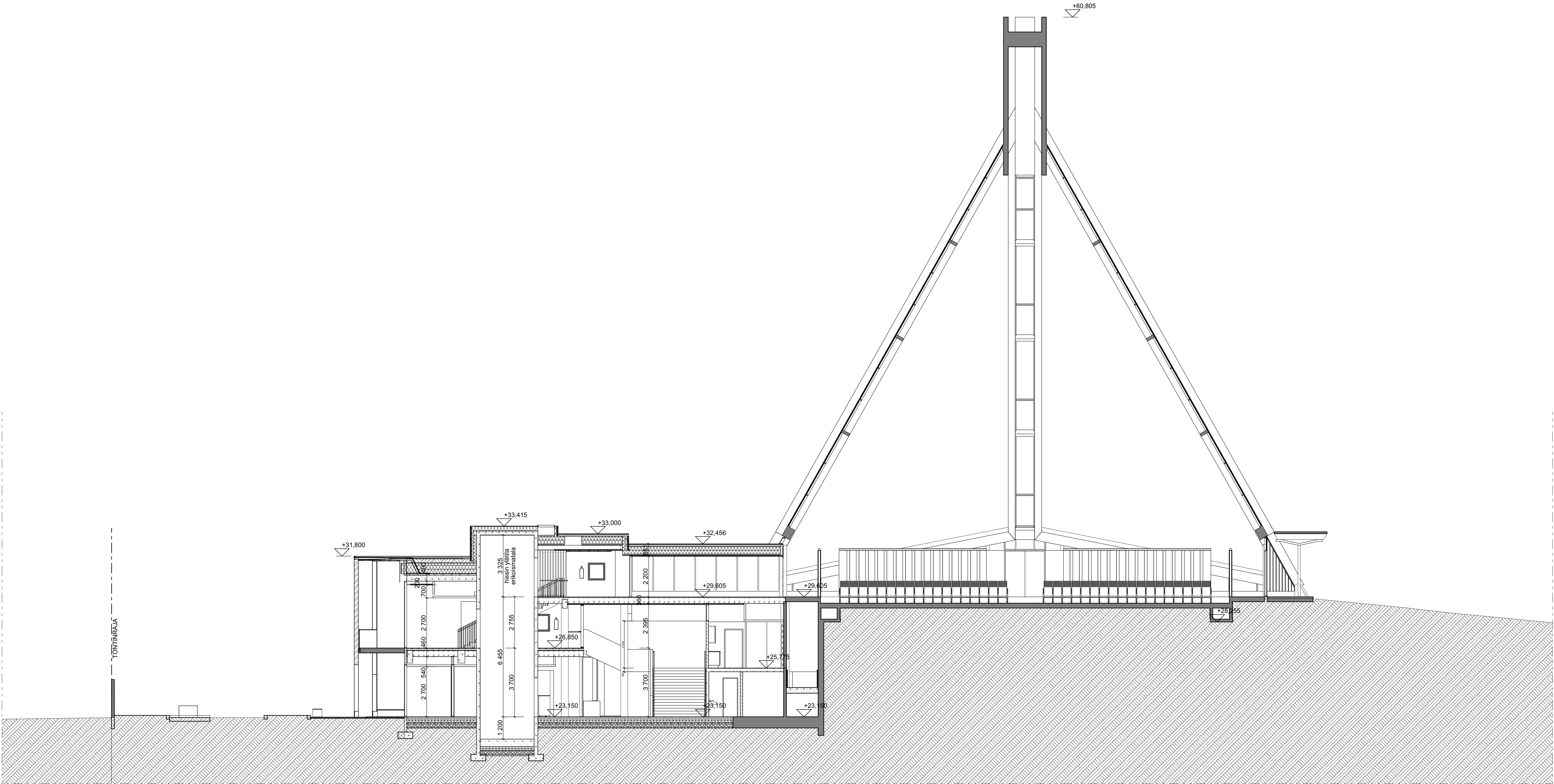
LEIKKAUS B-B
