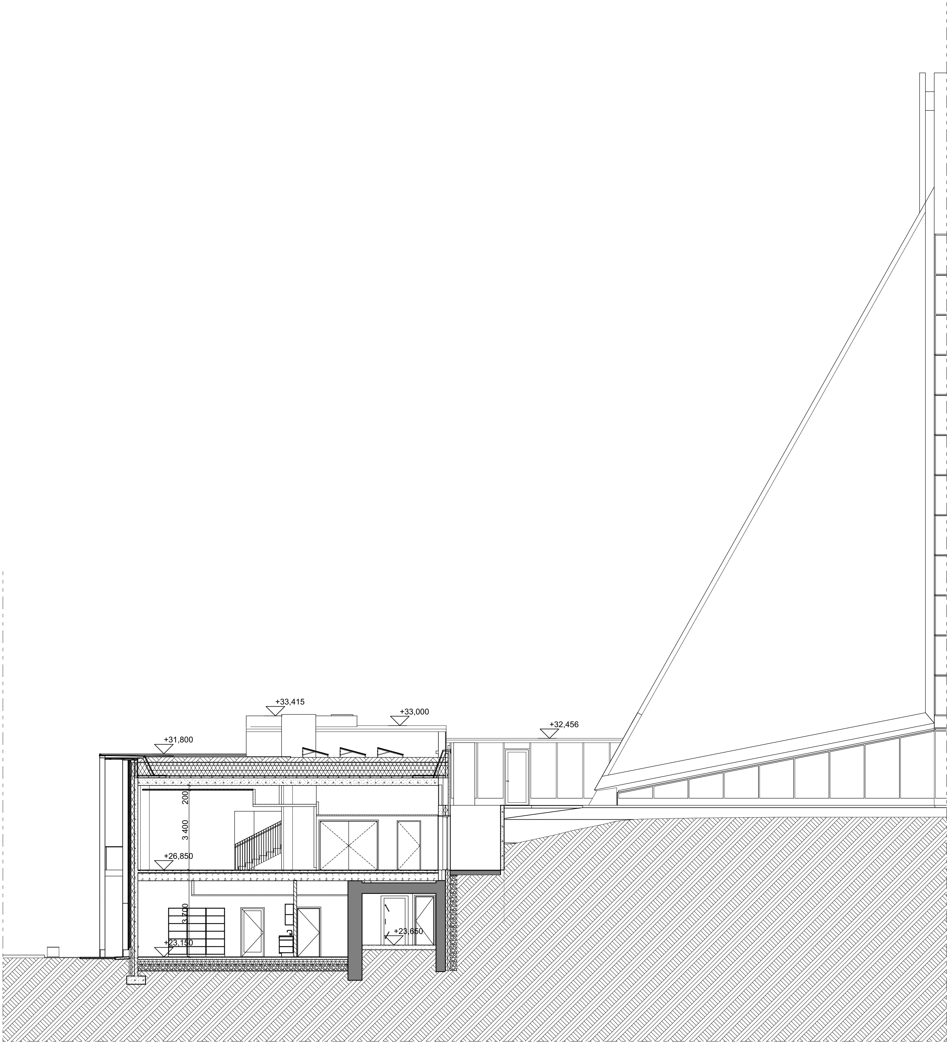
LEIKKAUS E-E
